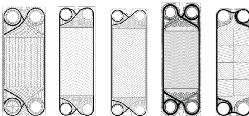
Thay gioăng tấm thiết bị trao đổi nhiệt DAEWON
